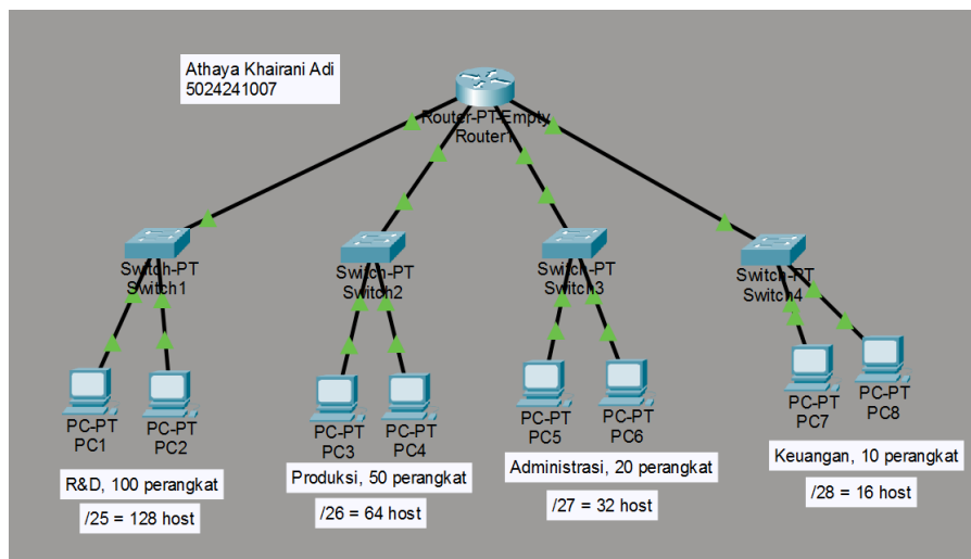
Gambar 1: Topologi LAN
